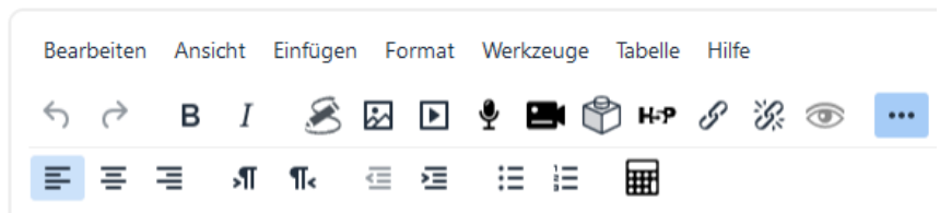
Abb. 2: TinyMCE Text-Editor
